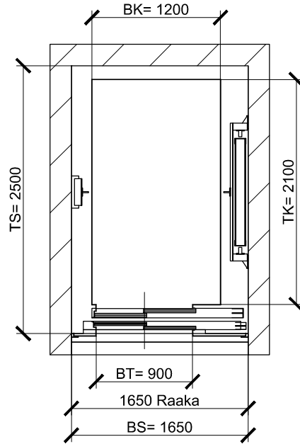
Korileikkaus 1:50
