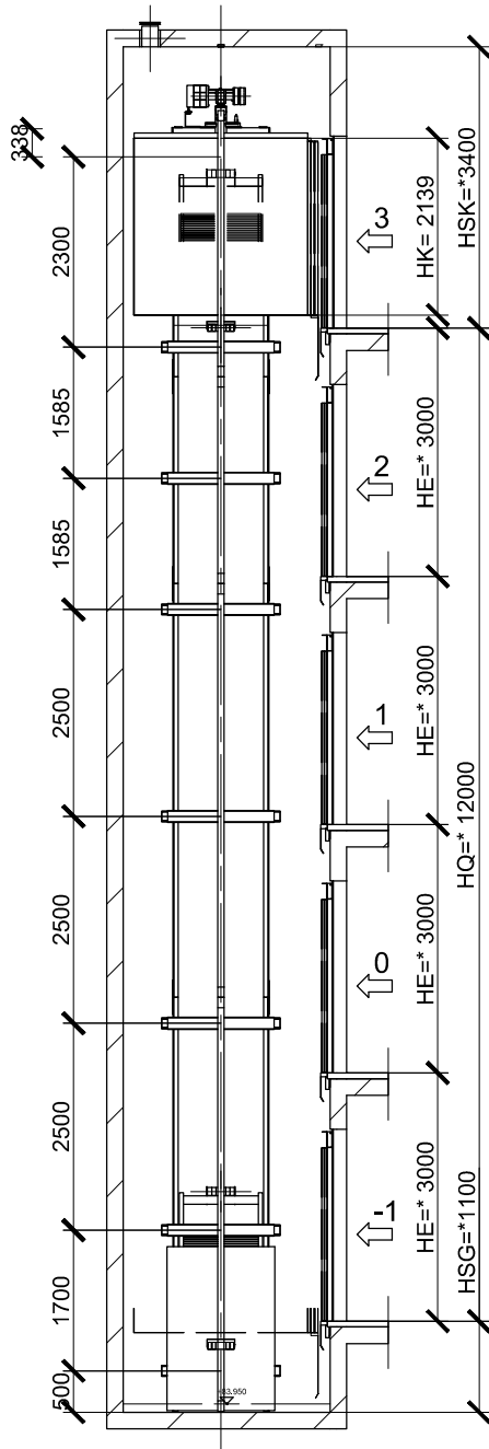
Pystyleikkaus 1:100
